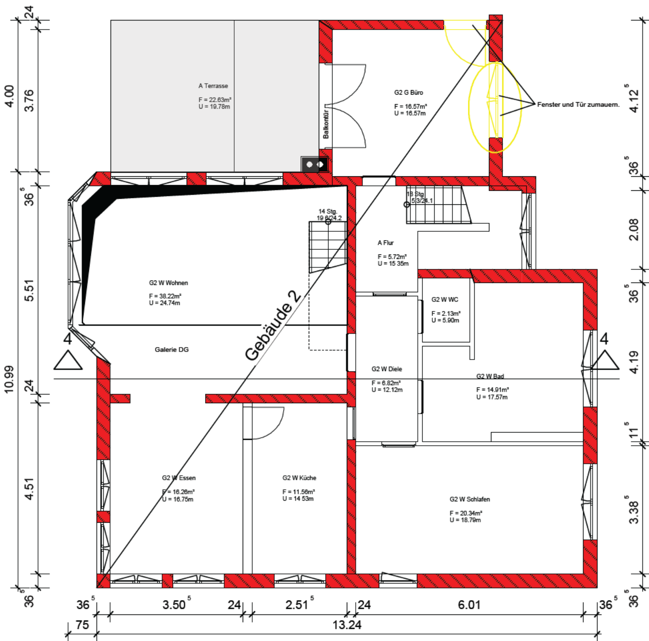
Grundriss Obergeschoß M1:100
