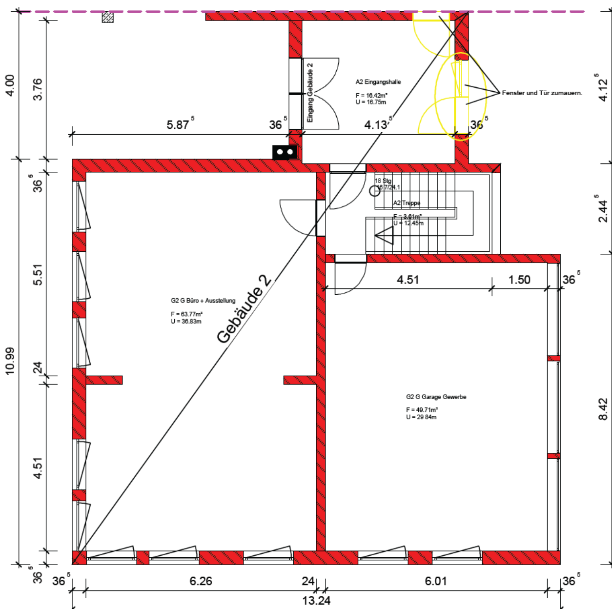
Grundriss Erdgeschoß M1:100
