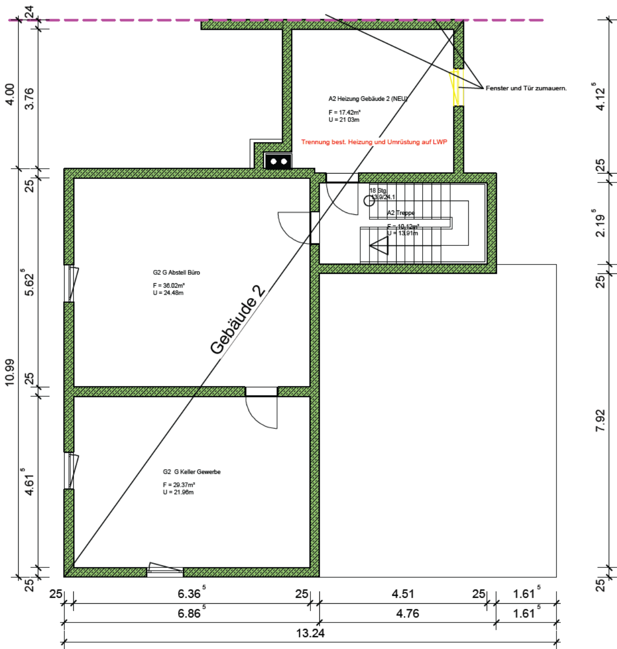
Grundriss Kellergeschoß M1:100
