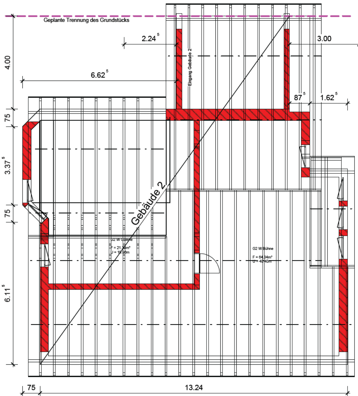
Grundriss Dachgeschoß M1:100
