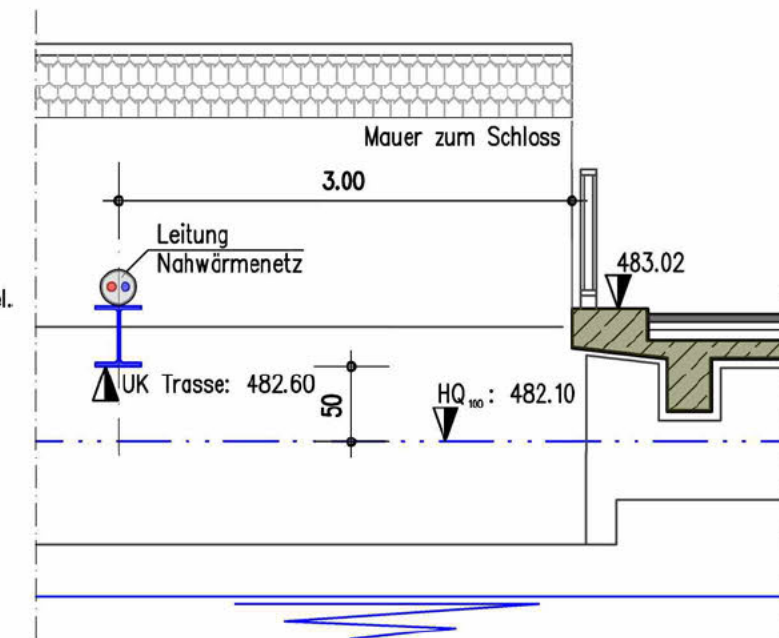
Schnitt "B-B"
