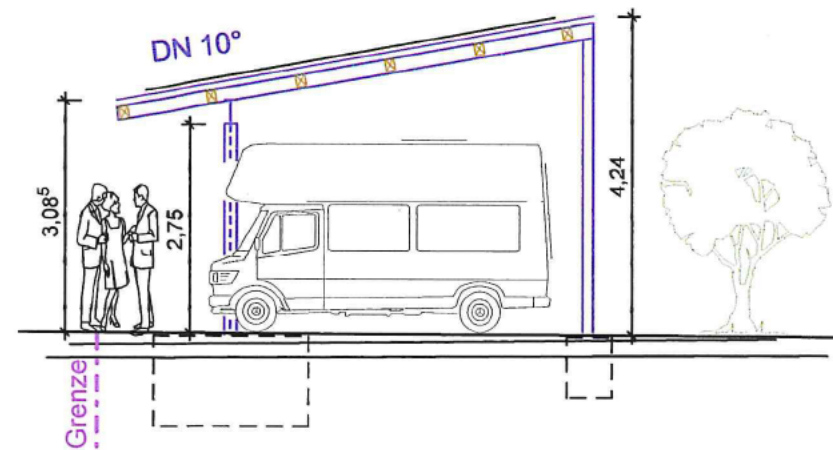
Ansicht West M1:100
