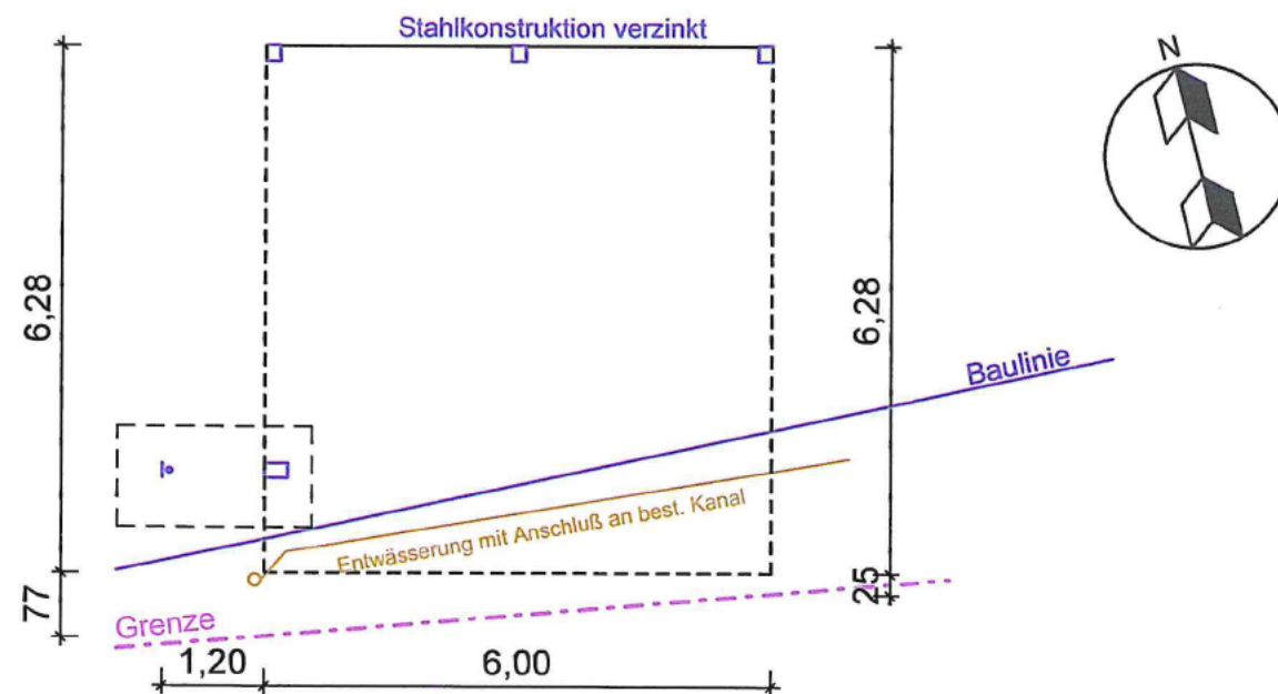
Grundriss M1:100
