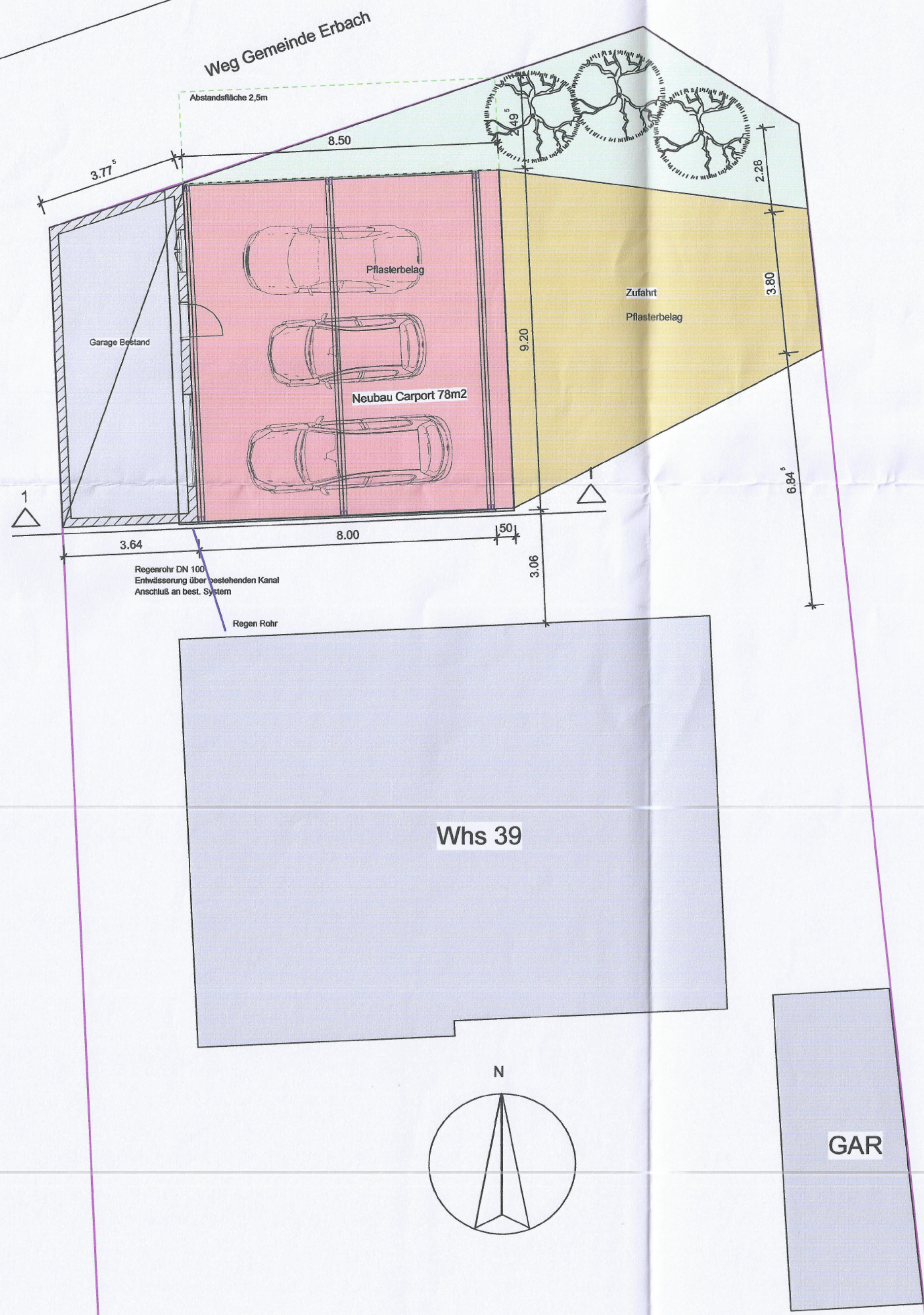
Grundriss EG M1: 100
