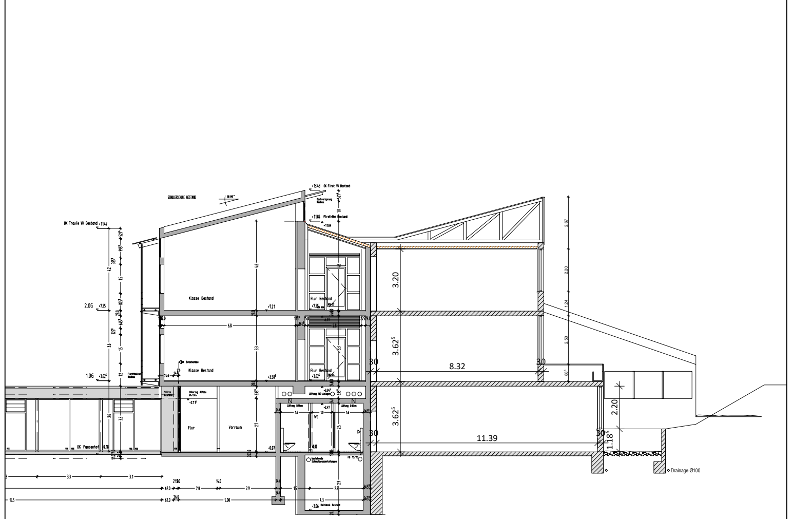
SCHILLERSCHULE Trakt I SCHNITT C-C BESTAND
