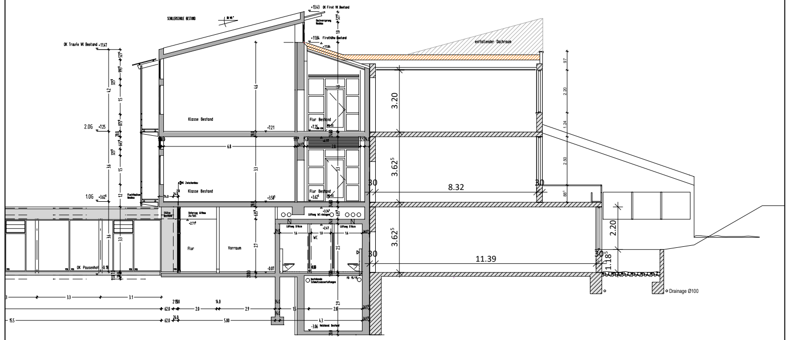
SCHILLERSCHULE Trakt I SCHNITT C-C NEU
