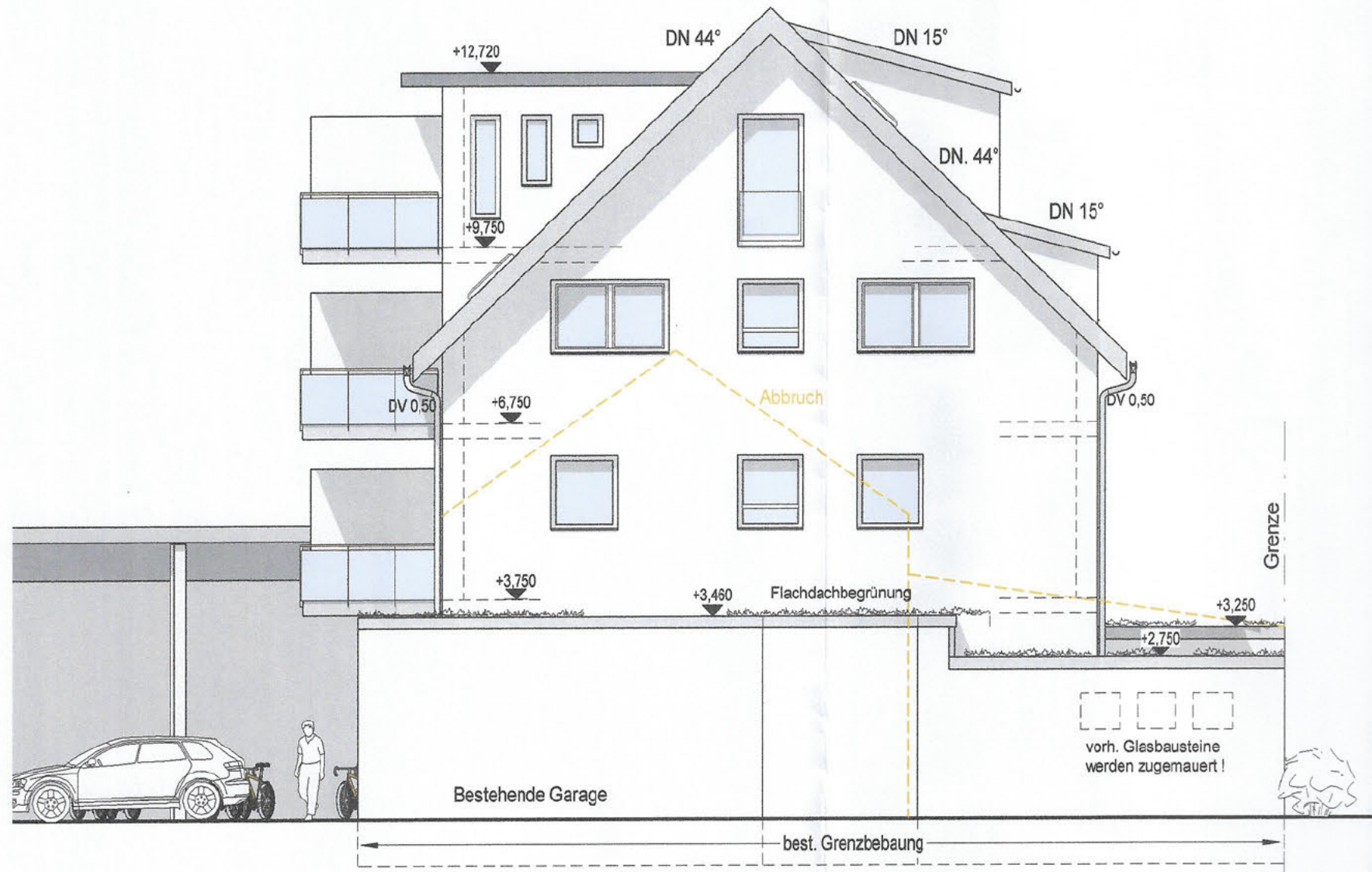
Südost M 1 : 100
