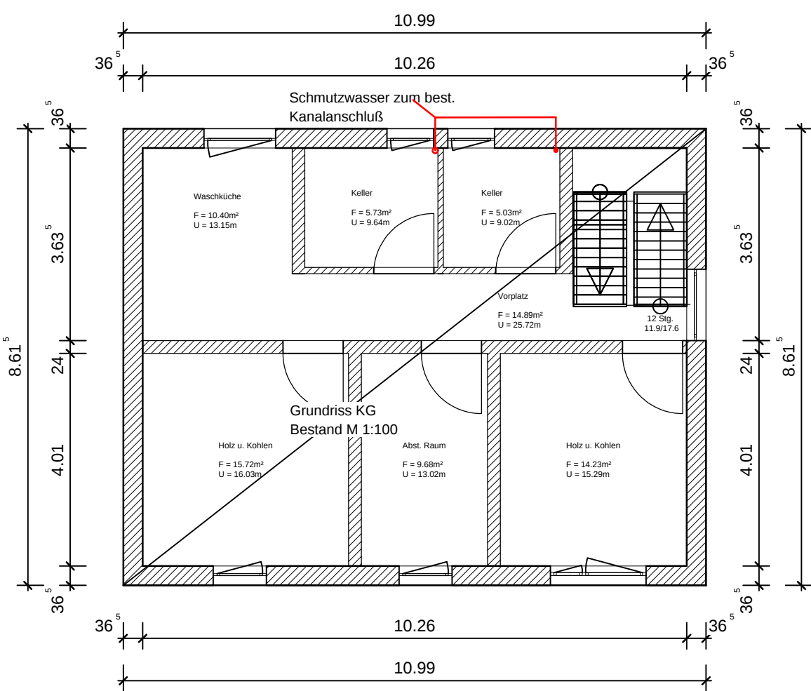
Grundriss KG M 1:100
