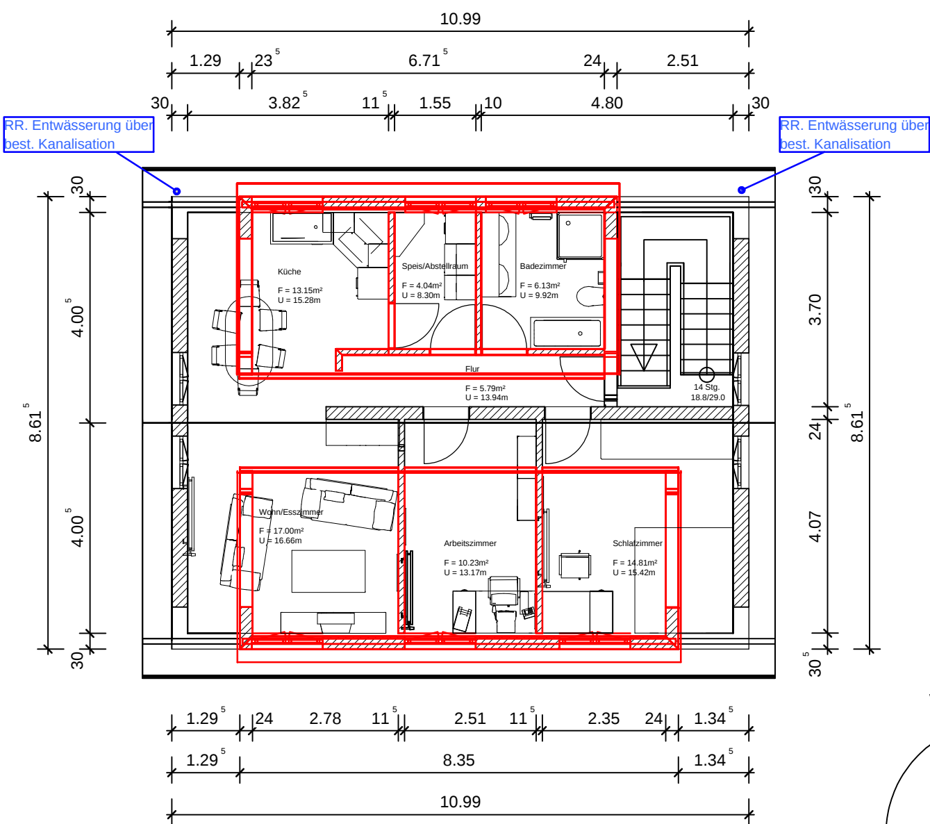
Grundriss DG M 1:100
