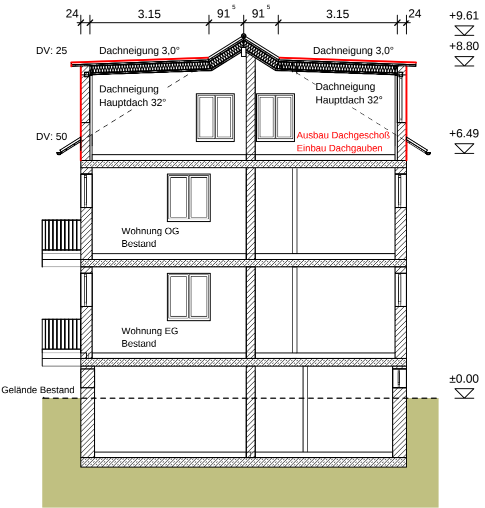
Schnitt M 1:100
