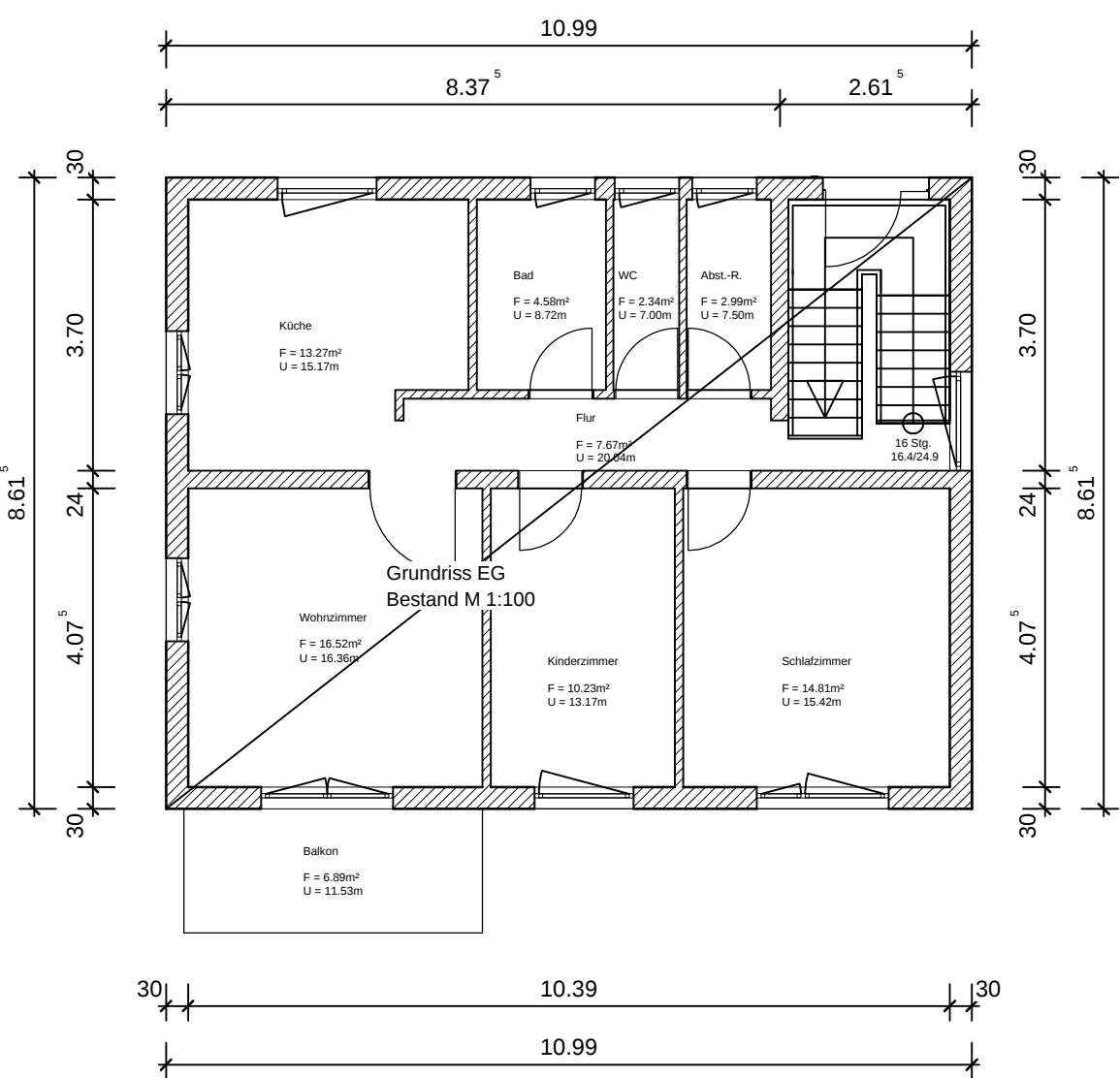
Grundriss EG M1:100
