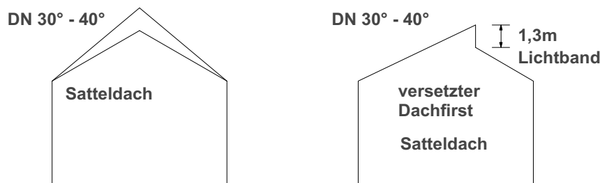
Skizze zur Dachform und Dachneigung
